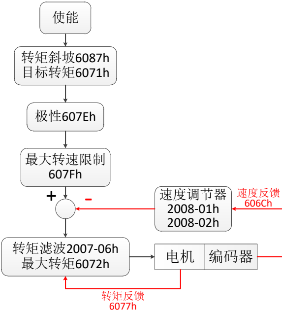
PT 模式控制框图
