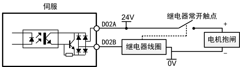
抱闸输出信号通过继电器控制电机抱闸
